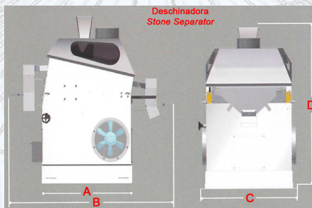
DIMENSIONES / SIZE (mm)
