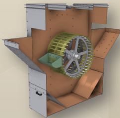
Dettalle elevador Detail elevator
